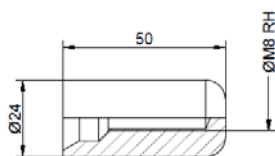
102244 M8 Rechtsgewinde Ms
