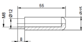
102204 M8 Messing
