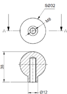
102203 M8 Kugel 32 Ms
