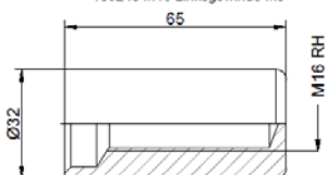
106239 M16 Rechtsgewinde Ms
