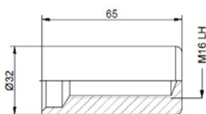
105876 M16 Linksgewinde Stahl
