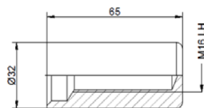
106240 M16 Linksgewinde Ms
