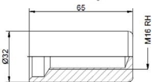
106239 M16 Rechtsgewinde Ms
