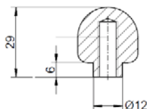
105869 M8 Kugel 25 Ms
